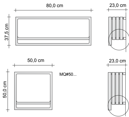
Posizione attacchi di allacciamento
